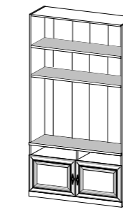
ME-9 panel RTV W: 2290 S: 1200 G: 410
