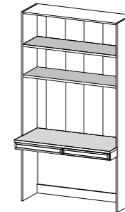
ME-7 panel z biurkiem W: 2290 S: 1200 G: 410/590
