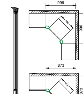
ME-słupek narożny \sphericalangle 45^\circ W: 2290 S: 52 G: 52
