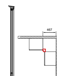
ME-słupek narożny \sphericalangle 90^\circ W: 2290 S: 67 G: 67
