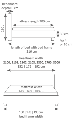
MINI MAXI bed with headboard 2300
