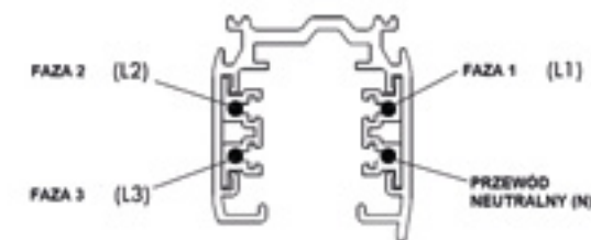
przekrój szyny track cross-section
