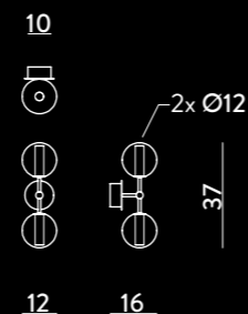
AP1571.2L APPLIQUE / WALL LAMP L 12 x 16 x H 37 cm G9 2 x max 33W 230V IP20
