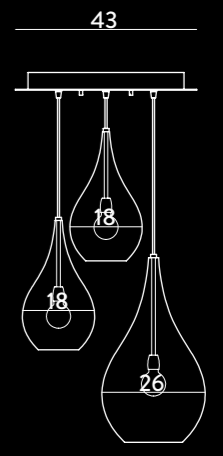
1259MX.3L PLAFONIERA / CEILING LAMP Glass Ø18/26 cm - cavo/cable 150 cm E14 2 x max 40W 220-240V E27 1 x max 70W 220-240V CE IP20 1m
