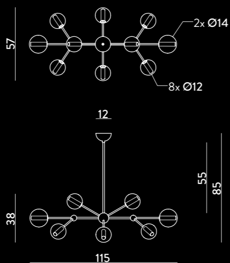
1574.10L LAMPADARIO / CHANDELIER L 115 - P 57 - H 85 cm G9 10 x max 33W 230V IP20
