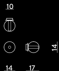
AP1571.14.1L APPLIQUE / WALL LAMP L 14 x 17 x H 14 cm G9 1 x max 33W 230V IP20
