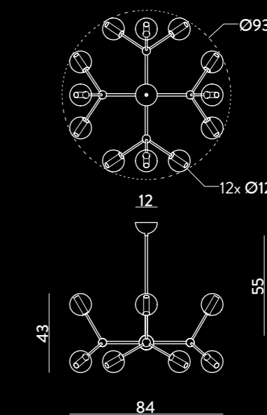
1574.12L LAMPADARIO / CHANDELIER Ø93 H 83 cm G9 12 x max 33W 230V IP20
