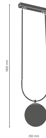
BALOS lampa wisząca 1 pł. 1 x E14/60W 0407 - czarno-złoty 0409 - biało-złoty
