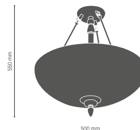
MODENA amplo 3 x E27, max 60W 729 - złoto 740 - chrom
