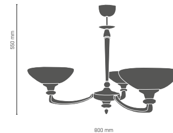
MODENA lampa wisząca 3 pł 3 x E27, max 60W 732 - złoto 743 - chrom
