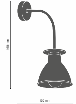
GAJA kinkiet 1 pt. 1 x E27, max 60W 0633 - złoty
