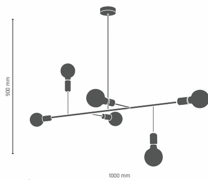
DADIM 6 x E27 max 60W 0192 - złoty
