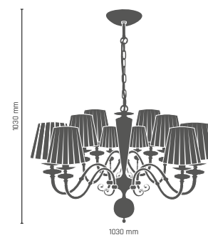
LILOSA lampa wisząca 10 pt. 10 x E14, max 60W 265 - złoto 228 - patyna połysk 274 - patyna mat 256 - chrom
