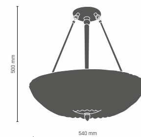
DIAMANTE ampla 3 x E27, max 60W 769 - złoto 793 - chrom 781 - patyna mat
