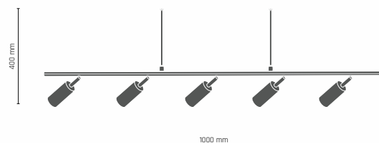
HUSO plafon 5 pt. 5 x GU10 35 mm, max 25W 0225 - czarno-złoty 0296 - biało-złoty
