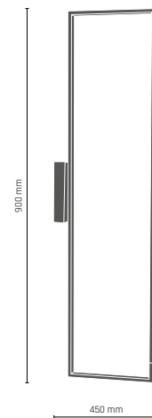
EBORA kinkiet listwa LED LLE FLEX G2 8 x 4800 12W 1800 lm/m 0648 - czarno-złota 0654 - biała-złota
