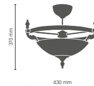
CORDOBA I plafon 3 x E27, max 60W 200 - patyna połysk 461 - patyna mat
