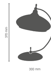
AGAT lampa nocna 1 x E27, max 60W 116 - złoto 107 - patyna połysk 431 - patyna mat
