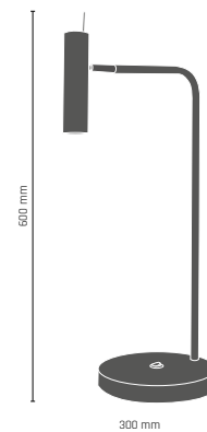
AMOS lampa gabinetowa. 1 x GU10 35mm / 25W 0174 - czarno-złoty 0177 - biało-złoty
