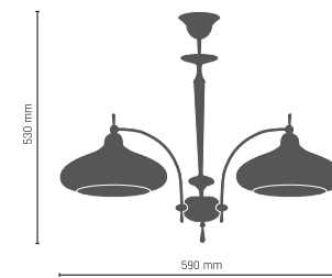
AGAT lampa wisząca 2 pt. 2 x E27, max 60W 113 - złoto 122 - patyna połysk 428 - patyna mat
