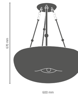
BUTTON ampla fi 60 6 x E27, max 60W 672 - złoto 677 - chrom
