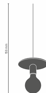
OLAIA lampa wisząca 1 x E27, max 60W 0522 - złota 0523 - patyna połysk 0524 - patyna mat
