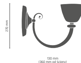
VERONA kinkiet 1 pł 1 x E27, max 60W 751 - złoto
