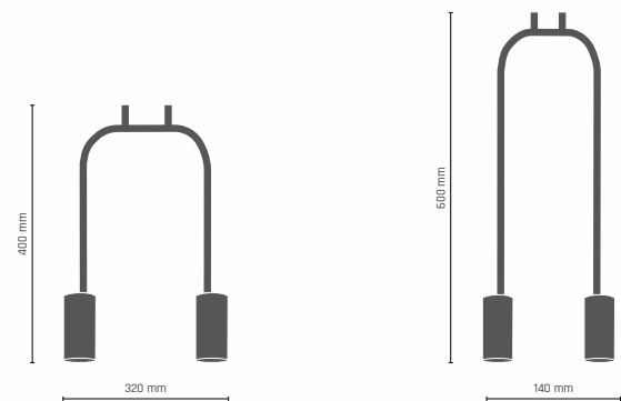
VAI lampa wisząca 2 pt. 2 x GU10 35 mm, max 25W 0289 - czarno-złota 0290 - biało-złota
