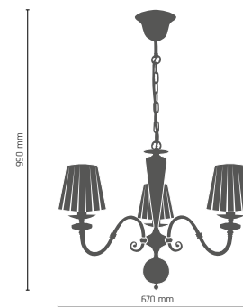
LILOSA lampa wisząca 3 pt. 3 x E14, max 60W 263 - złoto 226 - patyna połysk 272 - patyna mat 254 - chrom
