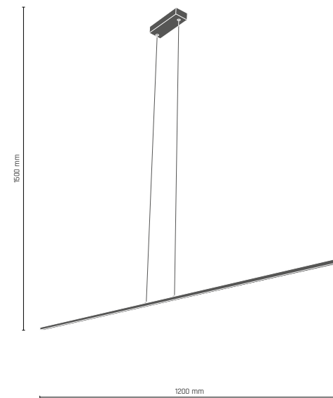
EBORA lampa wisząca listwa LED LLE FLEX G2 8 x 4800 12W 1800 lm/m 0644 - czarno-złota 0650 - biała-złota
