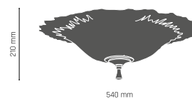
PLAFON II 3 x E27, max 60W 375 - złoto 366 - patyna połysk 418 - patyna mat
