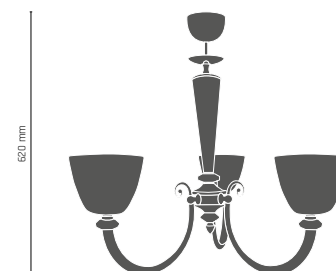
VERONA lampa wisząca 3 pł 3 x E27, max 60W 753 - złoto
