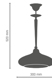
AGAT lampa wisząca 1 pt. 1 x E27, max 60W 112 - złoto 121 - patyna połysk 427 - patyna mat
