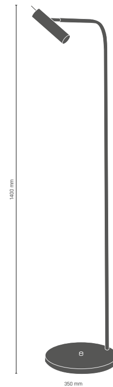
AMOS lampa gabinetowa. 1 x GU10 35mm / 25W 0175 - czarno-złoty 0178 - biało-złoty
