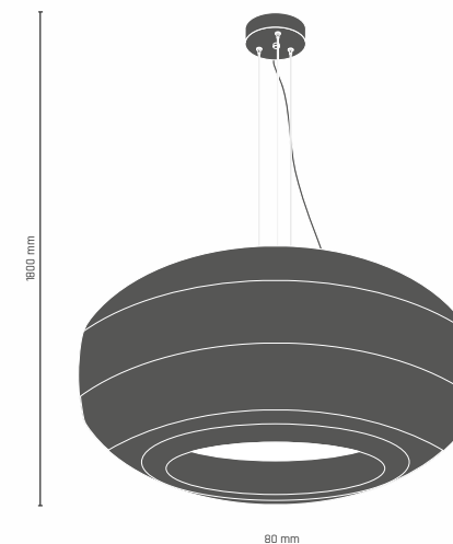
OLEDO lampa wisząca 1 p 6 x E27 / 9W LED 0221 - czarny 0222 - biały
