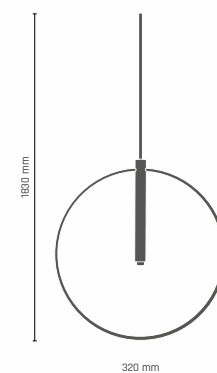
FARO lampa wisząca 1 pt. 1 x H-PIN 69 max. 20W 0553 - złoty
