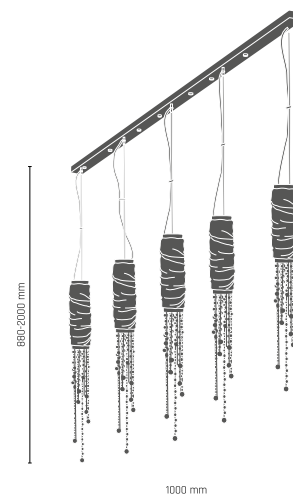
TUBO lampa wisząca 2 pt 2 x GU10/50W 407 - złoto 408 - chrom
