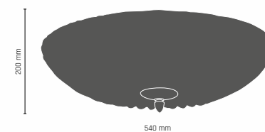
DIAMANTE plafon fi 54 3 x E27, max 60W 779 - złoto 803 - chrom 791 - patyna mat
