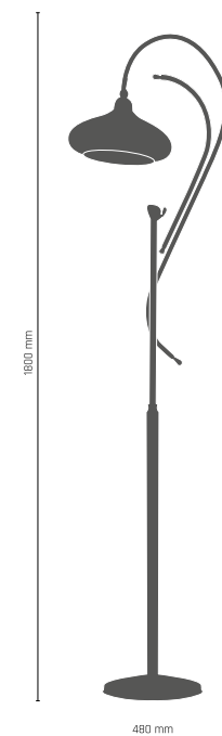
AGAT lampa podłogowa 1 x E27, max 60W 118 - złoto 127 - patyna połysk 433 - patyna mat
