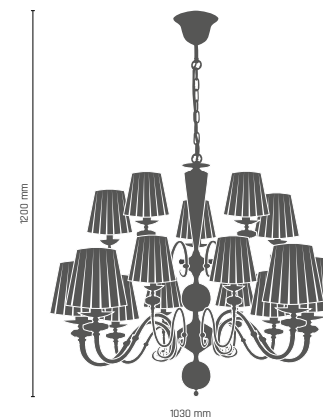
LILOSA lampa wisząca 15 pt. 15 x E14, max 60W 266 - złoto 229 - patyna połysk 275 - patyna mat 257 - chrom
