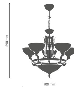
CORDOBA I lampa wisząca 3 pt. z ampla 3xE27, max 60W 3xE14, max 60W 195 - patyna połysk 456 - patyna mat
