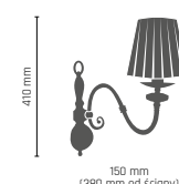
LILOSA kinkiet 1 pt. 1 x E14, max 60W 261 - złoto 224 - patyna połysk 270 - patyna mat 252 - chrom
