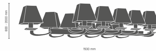
PLAZA listwa 12 pt. 12 x E14, max 40W 541 - złoto 555 - chrom
