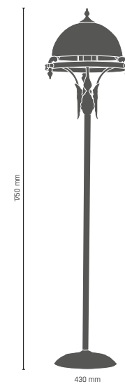
CORDOBA I lampa podłogowa 1 x E27, max 60W 199 - patyna połysk 460 - patyna mat
