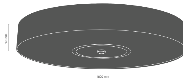
NABO plafon 100 10 x E27 / 9W LED 0282 - czarny 0286 - biały
