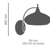
AGAT kinkiet 1 pt. 1 x E14, max 60W 111 - złoto 120 - patyna połysk 426 - patyna mat
