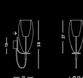
AP1391.1L Appique / Wall lamp vetro/glass Ø12 cm - cavo/cable 50 cm 💡 1 E14 x max 60W 220-240V C E IP20 (1m)
